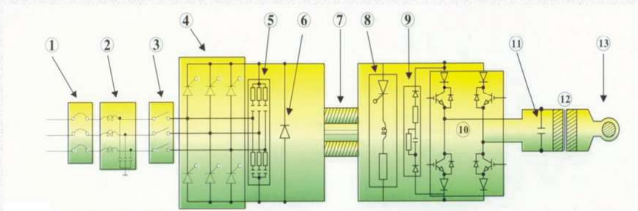
电气原理图 Schematic circuit diagram
